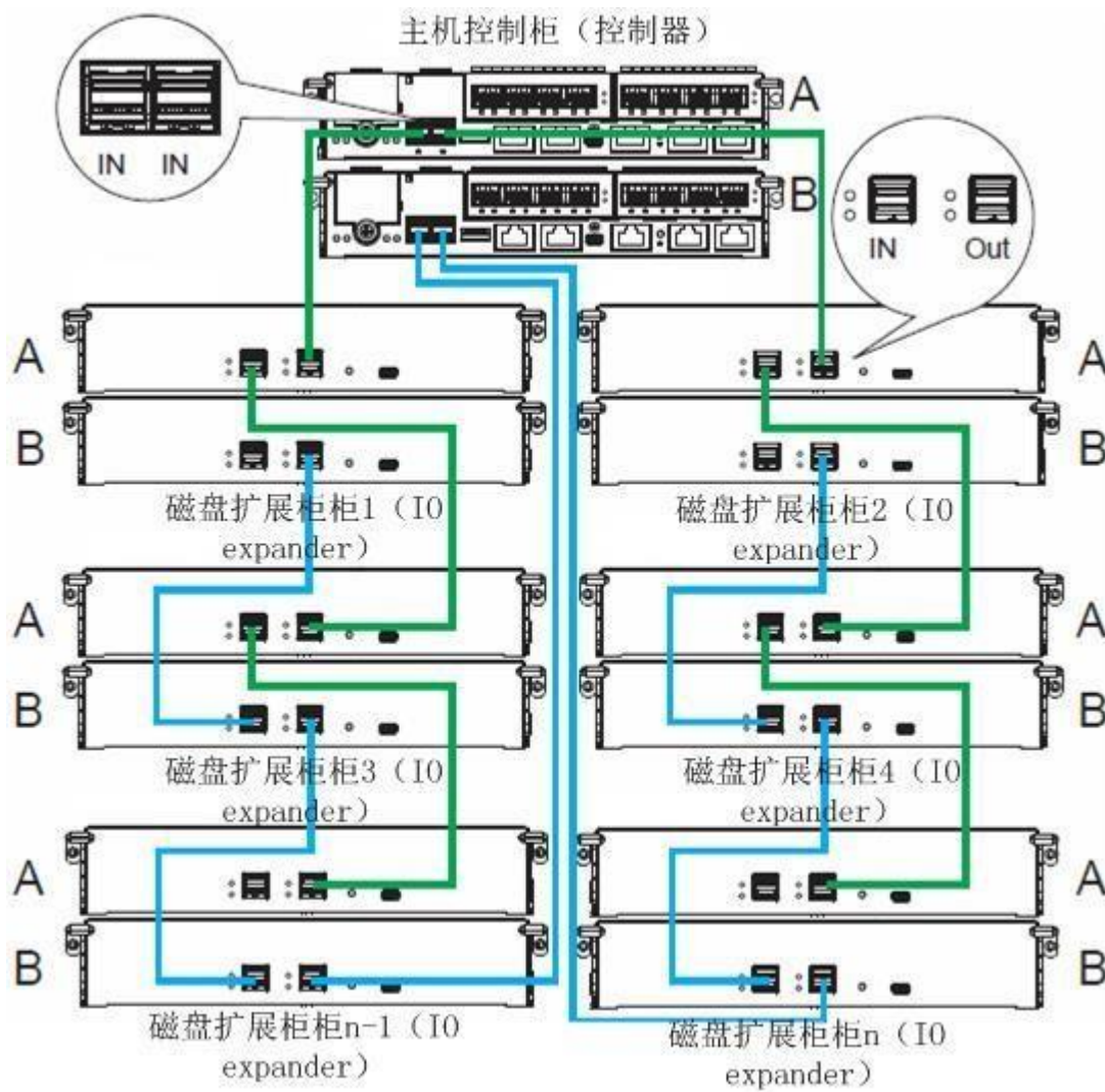
图 1- 7.GS6300X 扩展柜连接示意图
