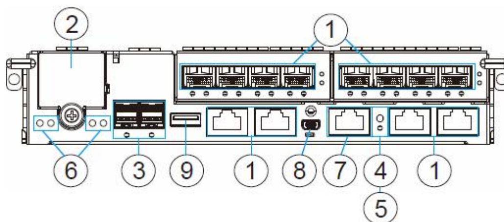
图 1- 6.控制器组成
