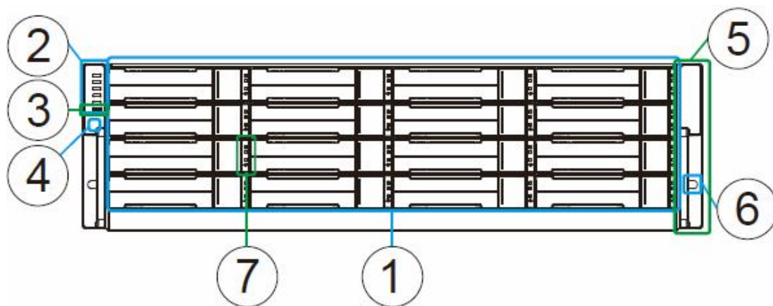
图 1- 3.GS6300X 前视图组件分布
