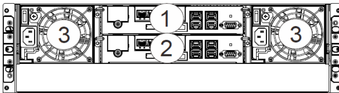
图 1- 4.GS6316D 后视图组件分布
