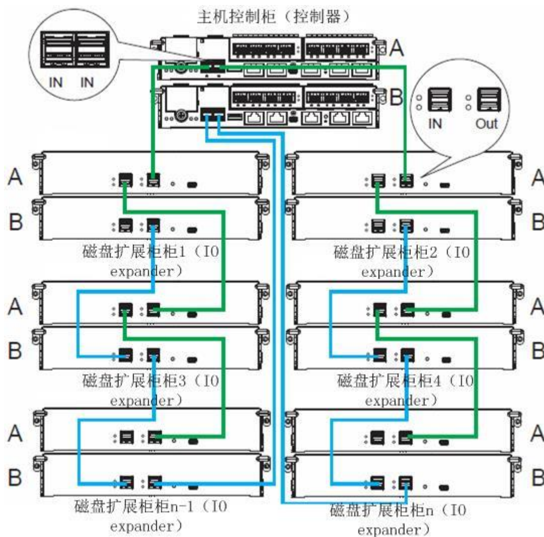
图 1-7.GS6316D 扩展柜连接示意图
