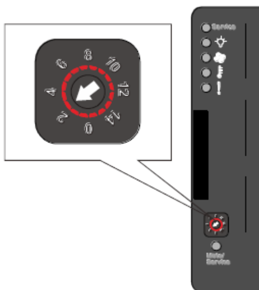
图 1-8.扩展柜 ID 设置
