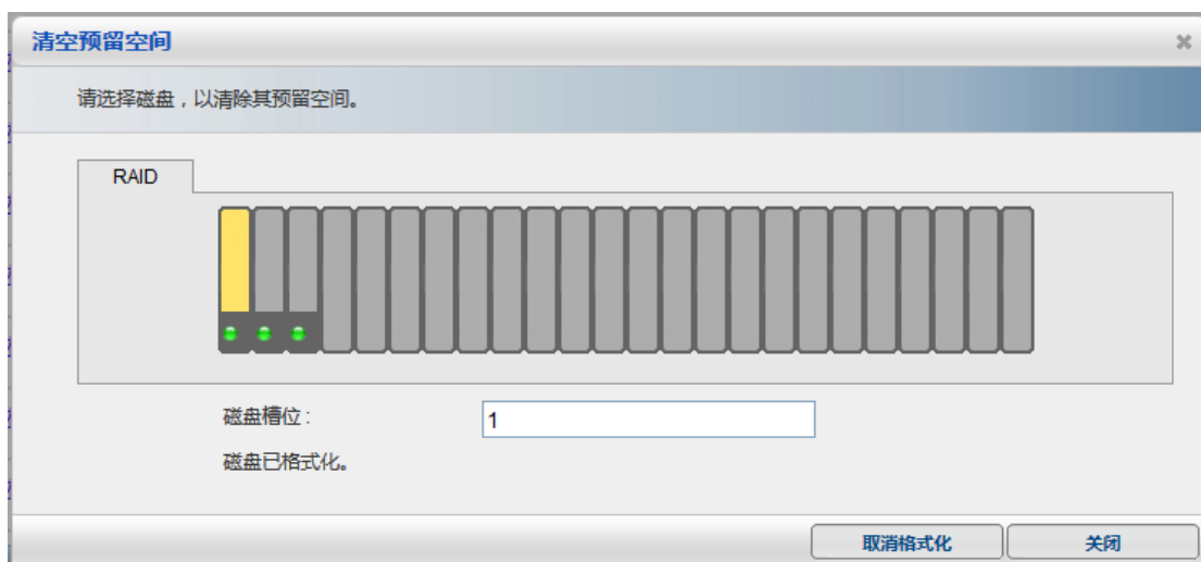
图 3- 73. 磁盘初始化
